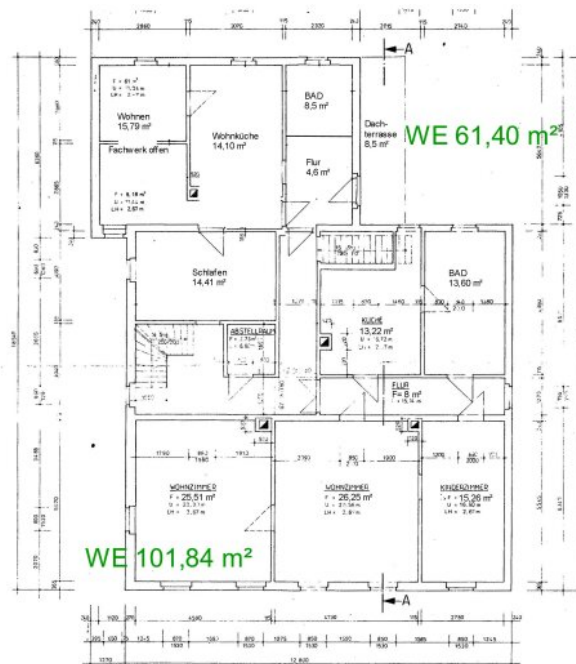
Grundriss DG
