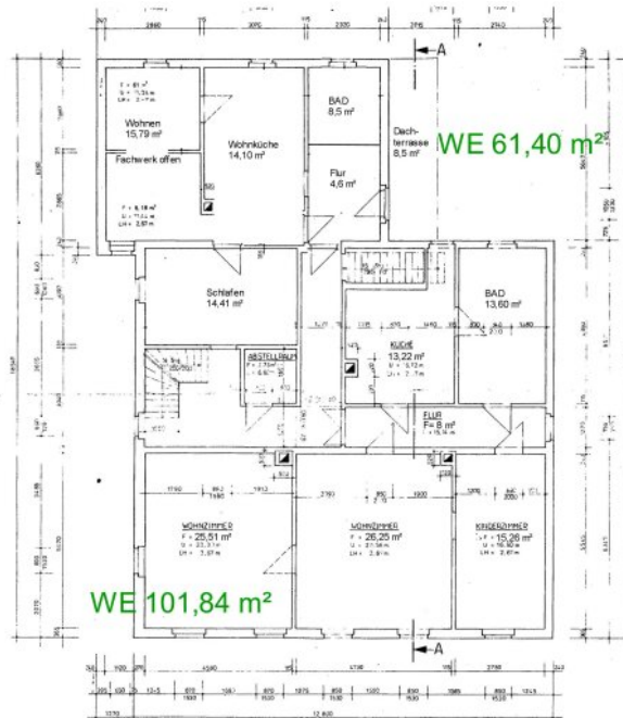
Grundriss DG
