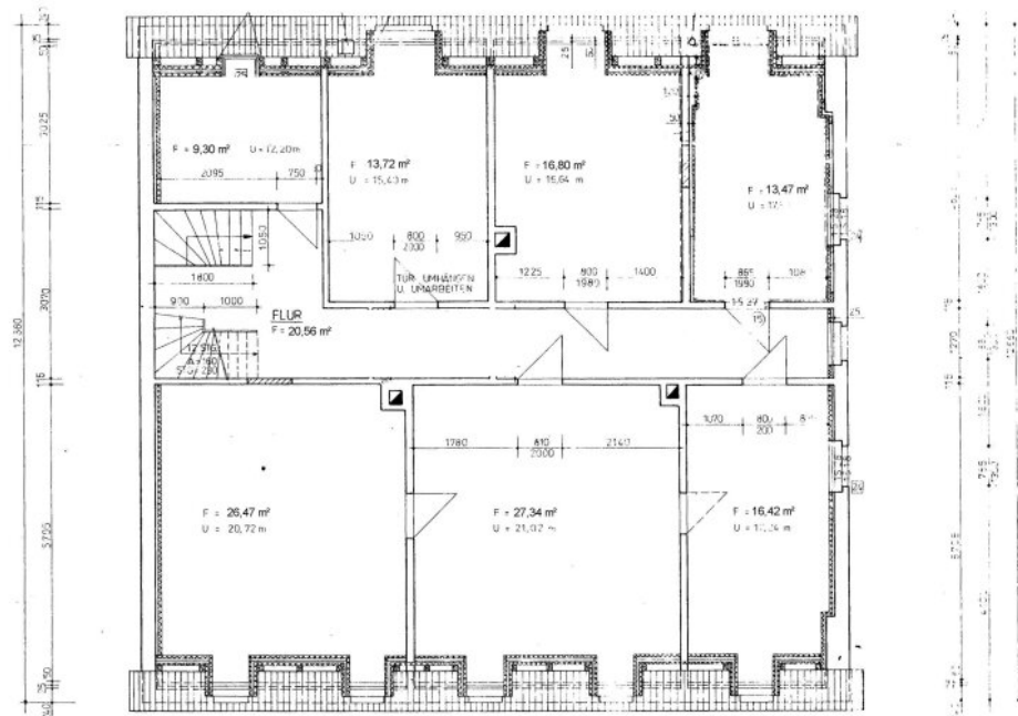
Grundriss DG
