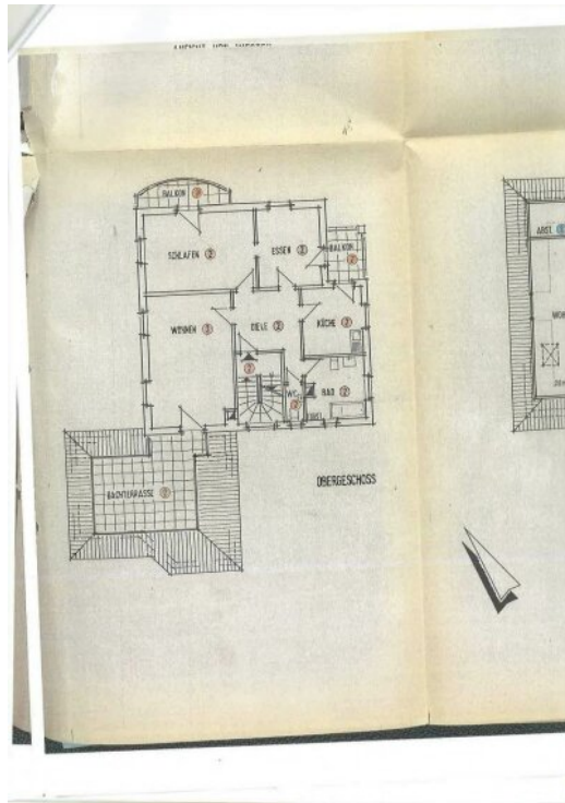
Wohnungsgrundriss Obergeschoss
