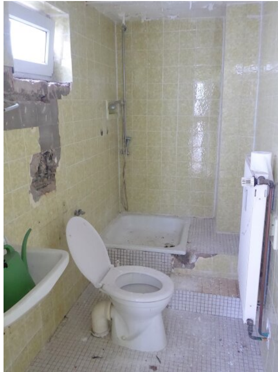
Duschbad vorne
