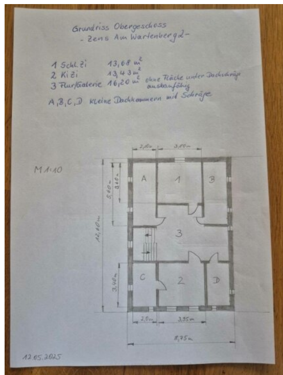
Grundriss DG
