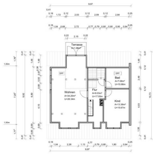
Grundriss DG
