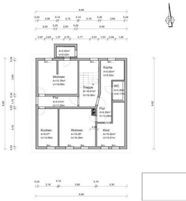
Grundriss OG
