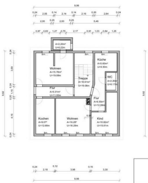
Grundriss OG
