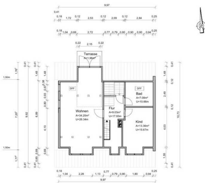
Grundriss DG
