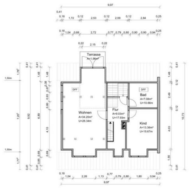
Grundriss DG
