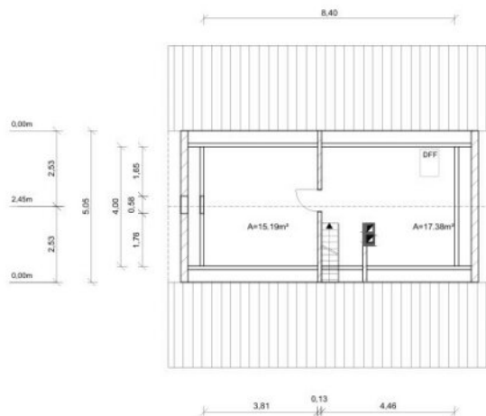
Grundriss Dachboden
