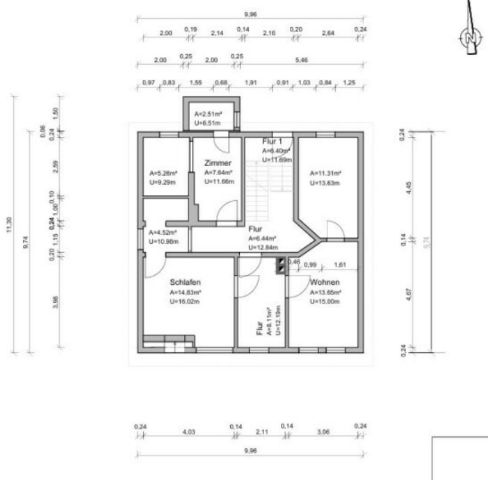
Grundriss EG
