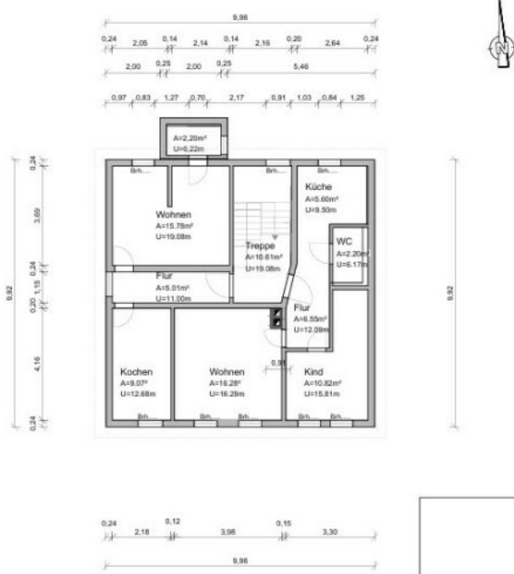
Grundriss OG
