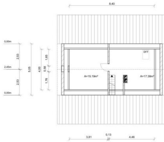
Grundriss Dachboden
