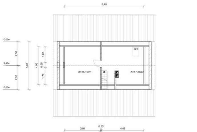
Grundriss Dachboden
