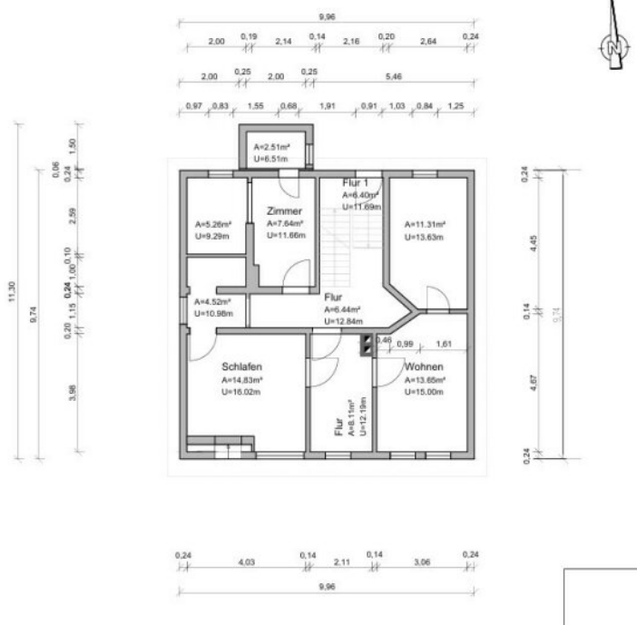
Grundriss EG
