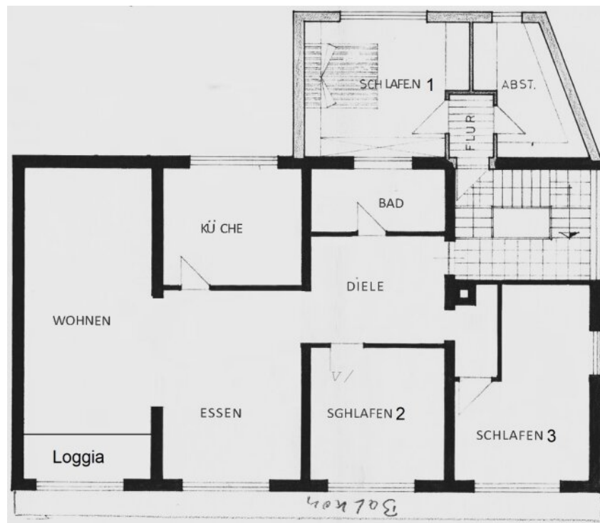
Grundriss Obergeschoss
