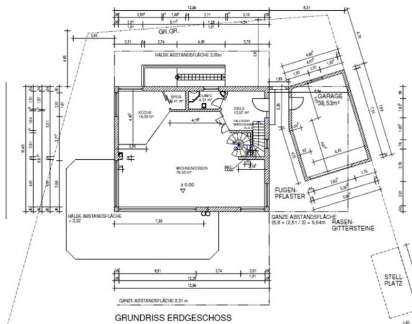
Grundriss Erdgeschoss
