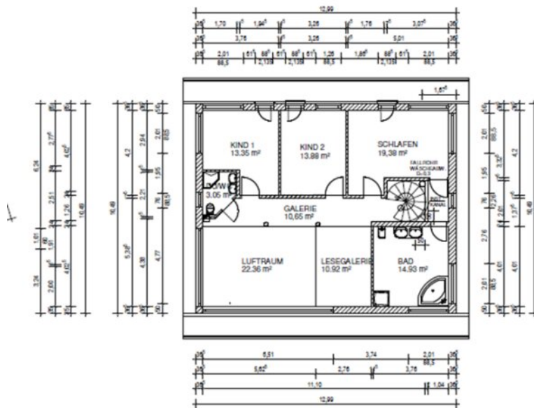
GRUNDRISS OBERGESCHOSS
