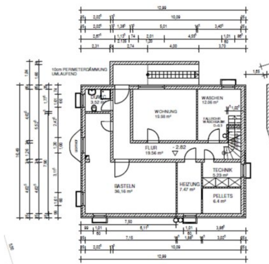
GRUNDRISS KELLERGESCHOSS
