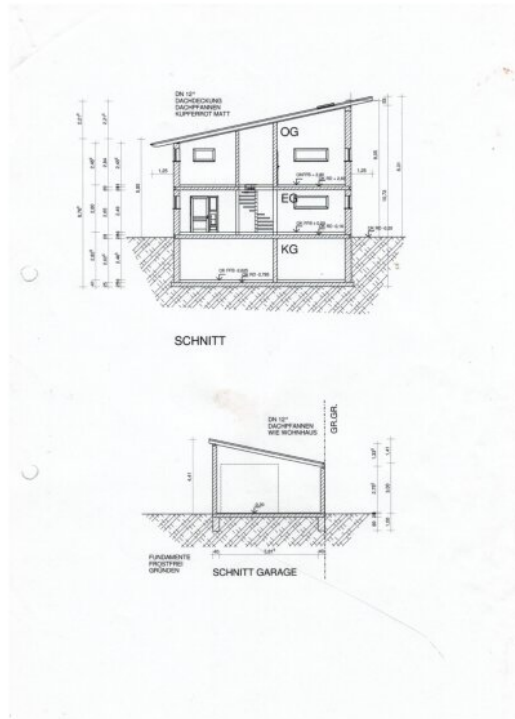
Schnitt
