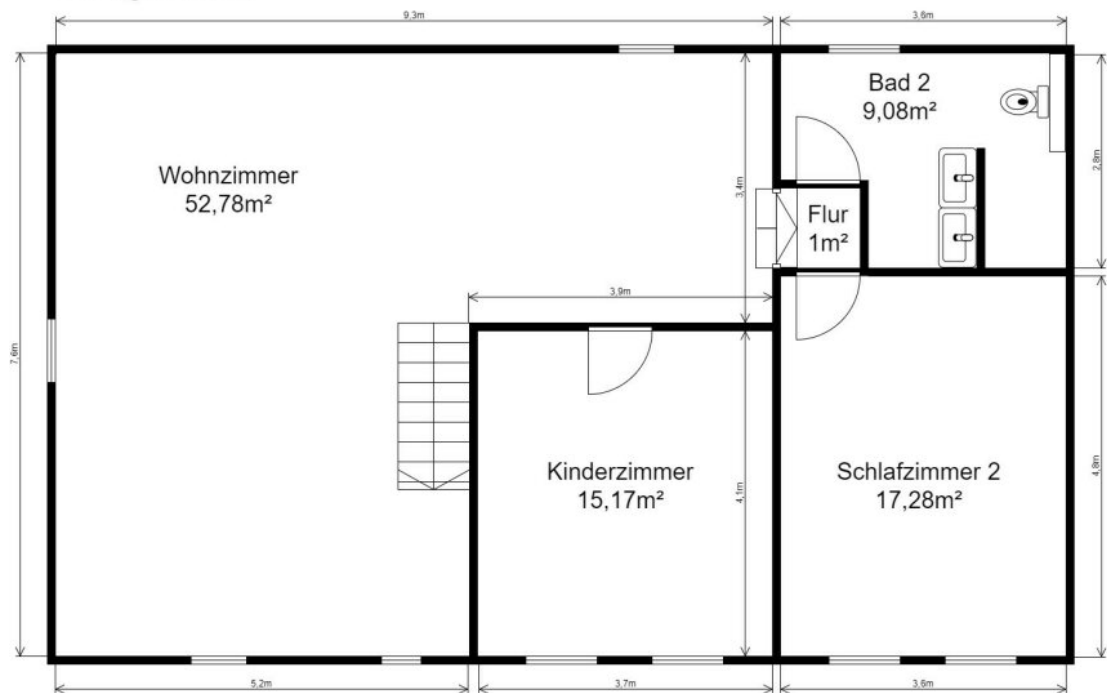
Grundriss OG
