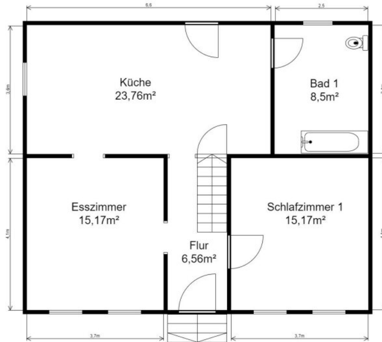
Grundriss EG
