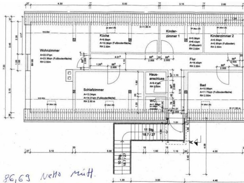
Grundriss DG-Planung
