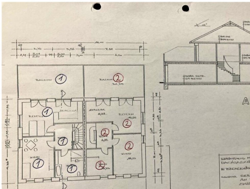
Grundriss OG
