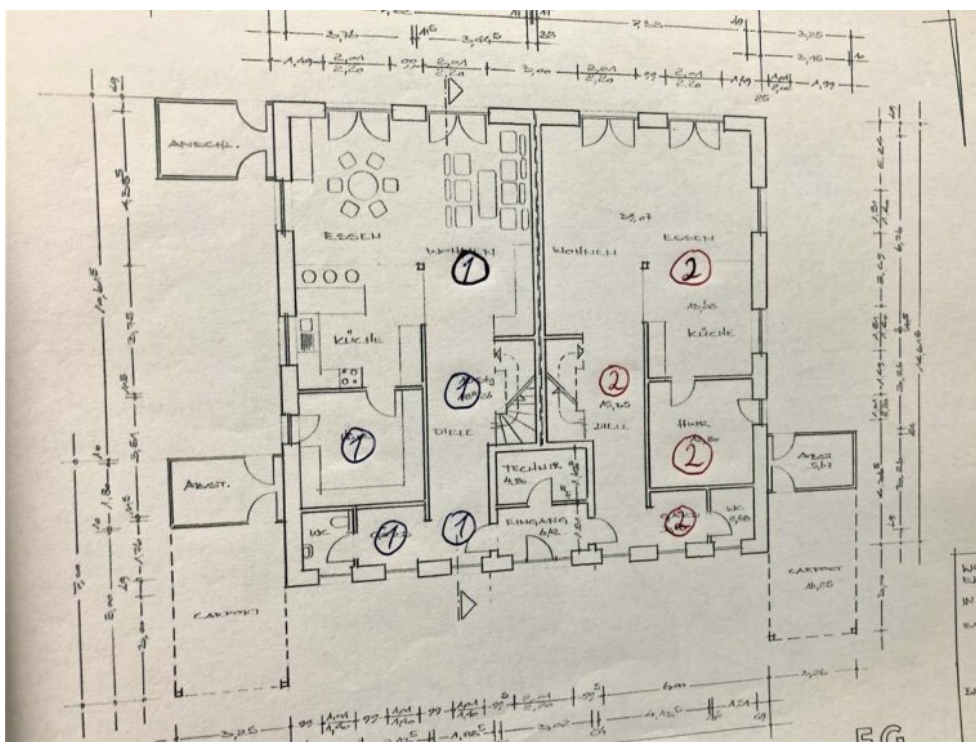
Grundriss EG
