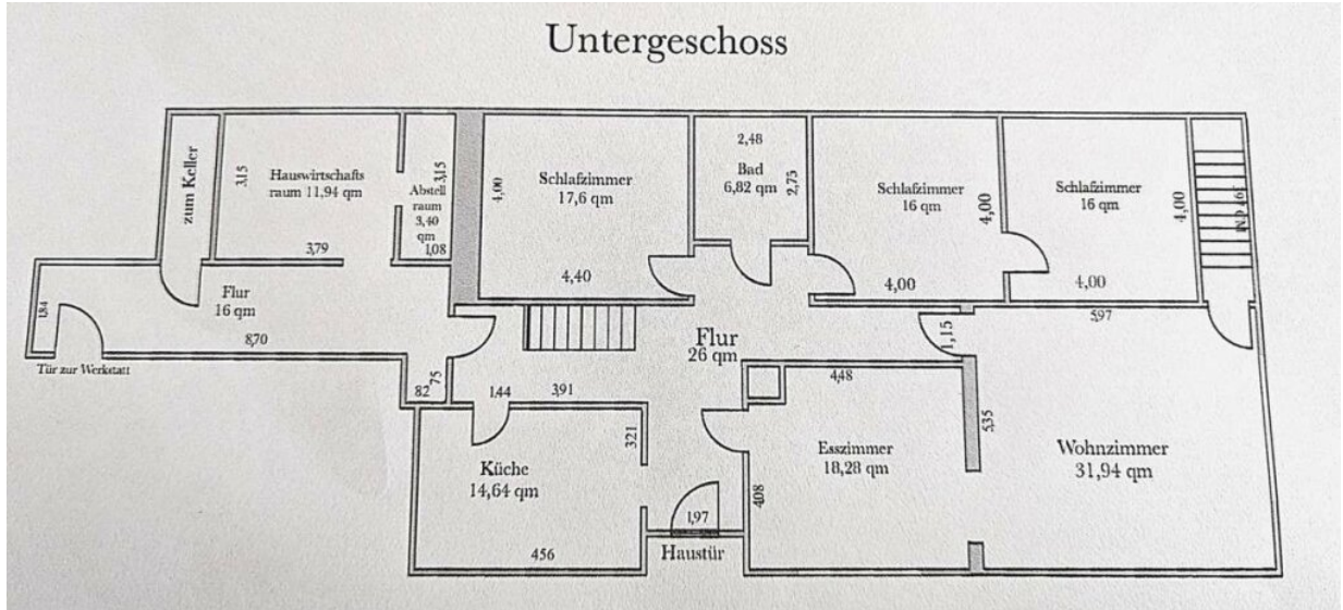
Grundriss UG Wohnhaus
