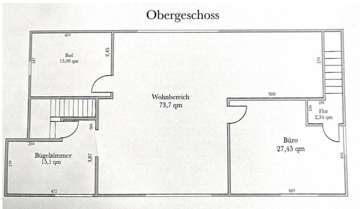
Grundriss OG Wohnhaus
