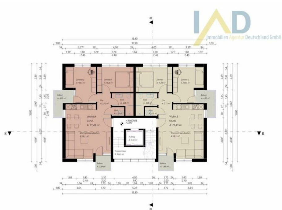
Grundriss Erdgeschoss
