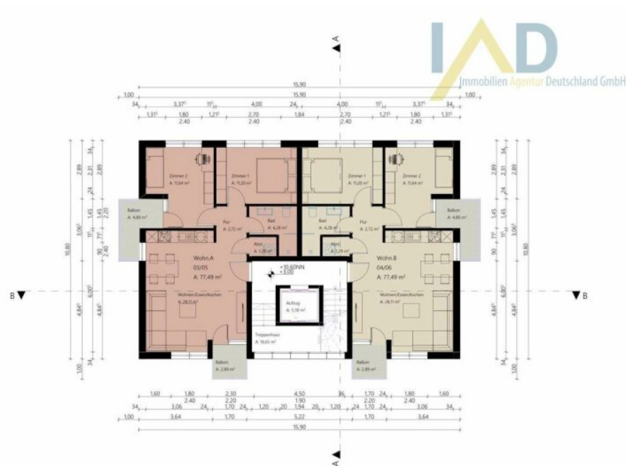
Grundriss Erdgeschoss
