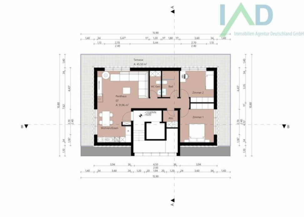
Grundriss Staffelgeschoss
