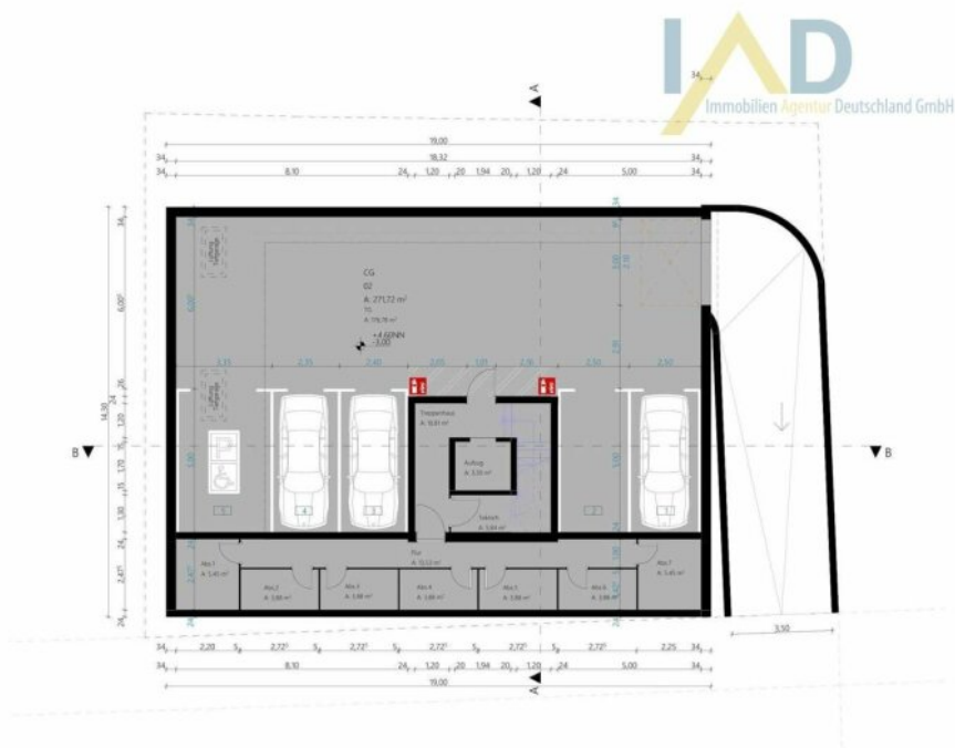
Grundriss Tiefgarage-1
