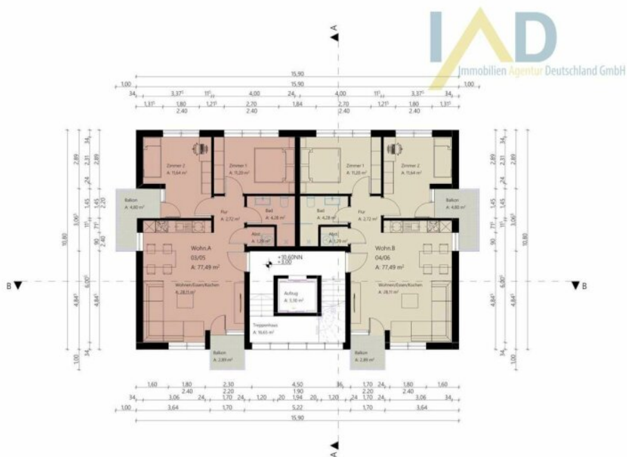
Grundriss OG-1
