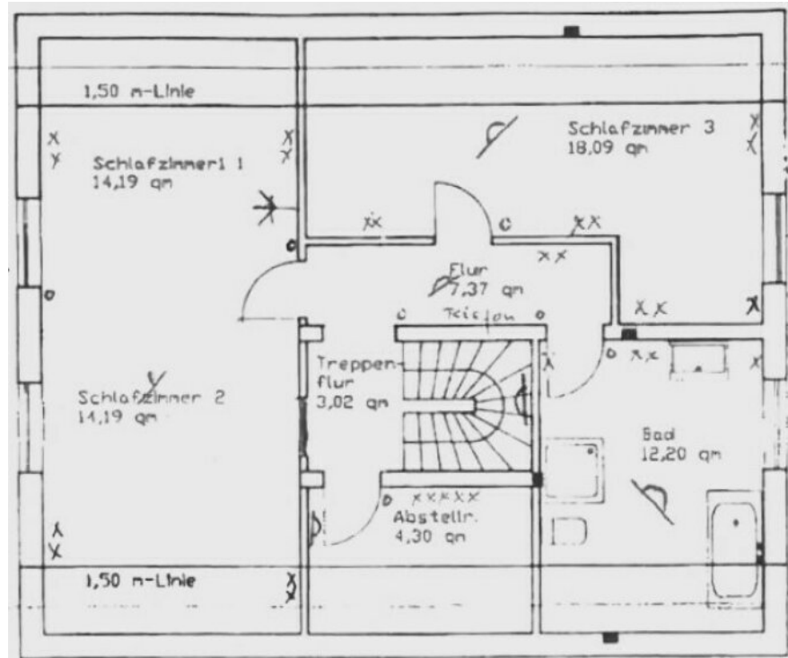
Grundriss DG
