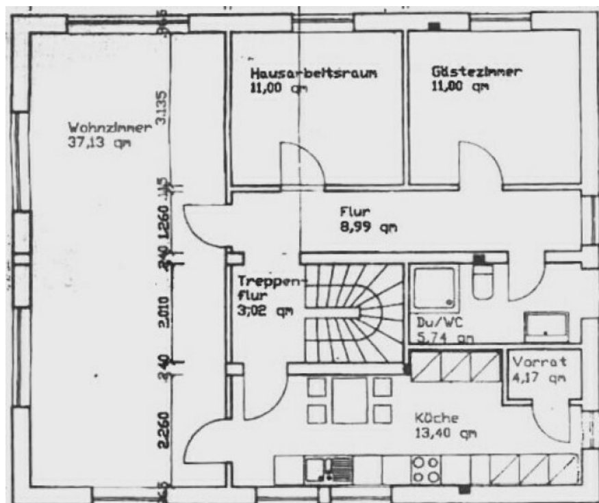
Grundriss OG
