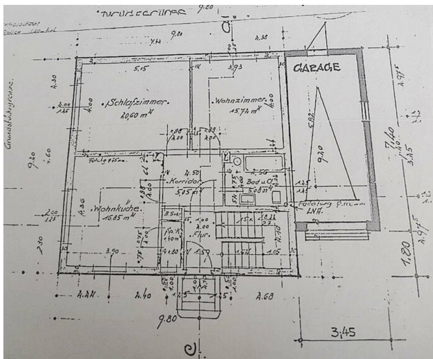
Grundriss EG
