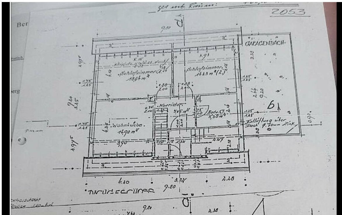
Grundriss OG
