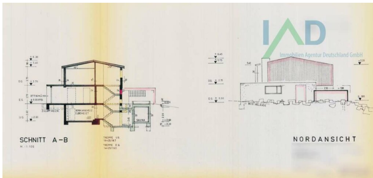
Nordansicht
