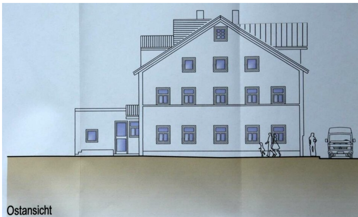
Ansicht Ost
