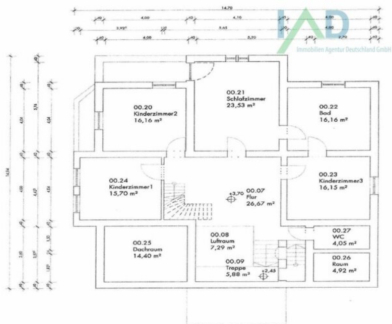
Grundriss Obergeschoss
